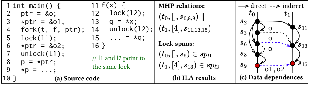
Fig. 10. FSPTA slicing example.
